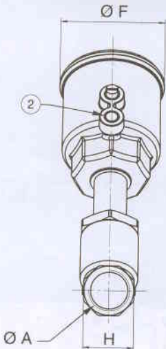
63,90和125mm气控头
