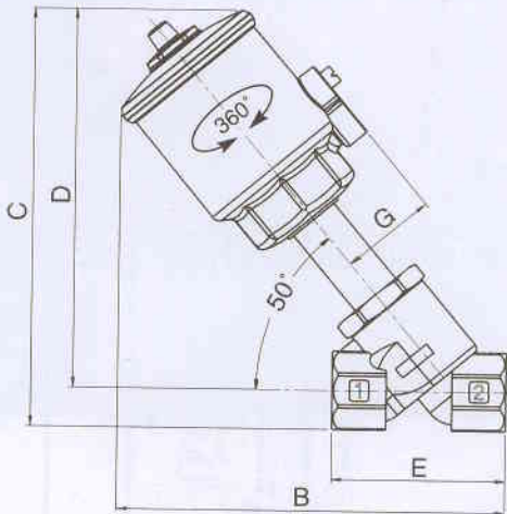
带90mm气控头结构
